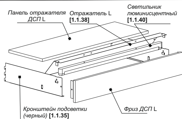
Панель отражателя ДСП L
